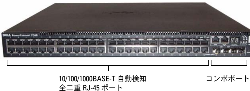
図 1-4. 10/100/1000BASE-T ポートを 48 個備えた PowerConnect 7048
