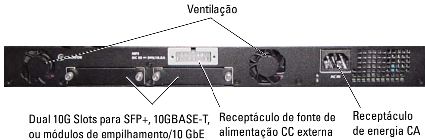
Figura 1-9. Pannel traseiro do PC7024P e PC7048P
